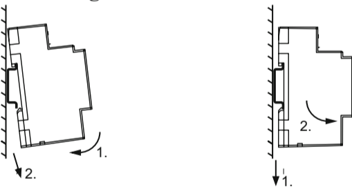
Abbildung 1: Montage
