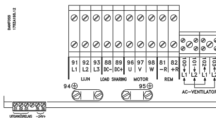
Afbeelding 8 Compact IP 54 5016-5062, 380-500 V 5008-5027, 200-240 V
