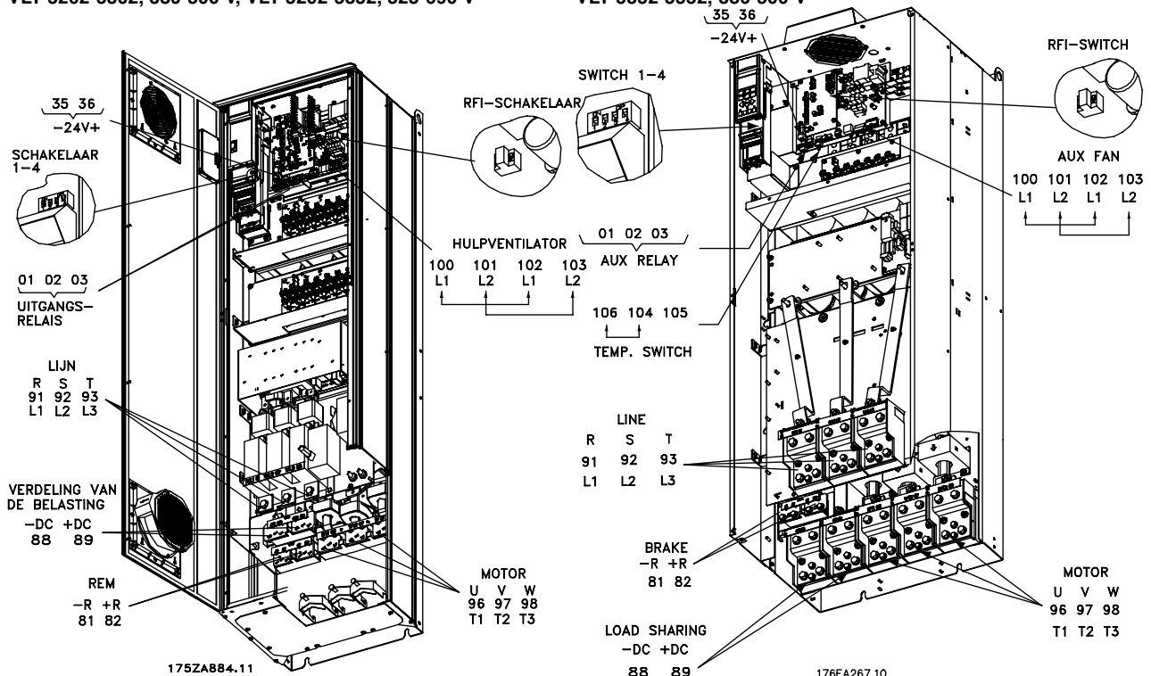
Compact IP 21/IP 54 met lastschakelaar en zekering VLT 5202-5302, 380-500 V, VLT 5202-5352, 525-690 V
