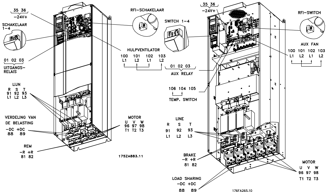
Compact IP 00 met lastschakelaar en zekering VLT 5202-5302, 380-500 V, VLT 5202-5352, 525-690 V
