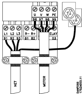
Afbeelding 5 Bookstyle IP 20 5001-5011, 380-500 V 5001-5006, 200-240 V
